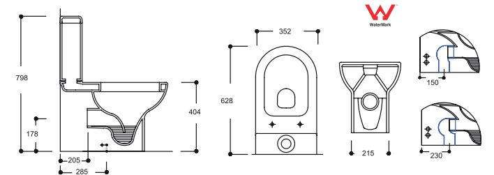
K005KLZ00 COMPACT DUVARA DAYALI KLOZET K001RZV00 REZERVUAR K000KRK48 KLOZET + REZERVUAR
