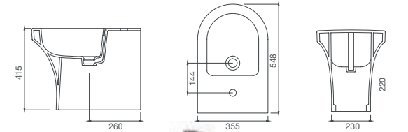
SO02BDE00 SOLE DUVARA ASMA BIDE
