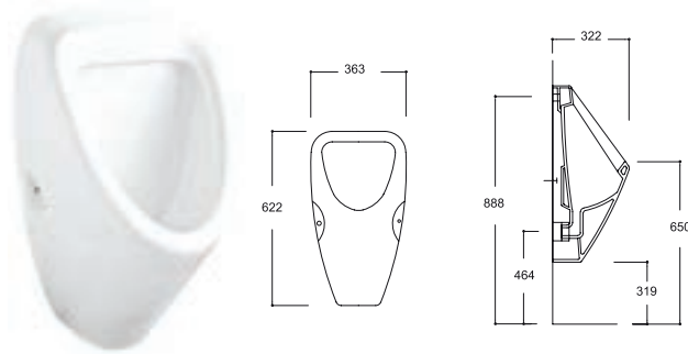
TP04PSR00 | TP04PSR00 FOTOSEL UYUMLU PİSUVAR | URINAL
