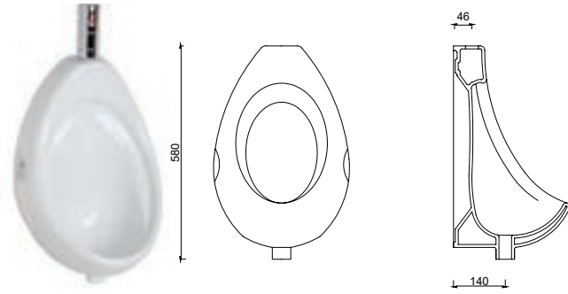
TP07PSR00 | TP07PSR00 FOTOSEL UYUMLU PİSUVAR | URINAL
