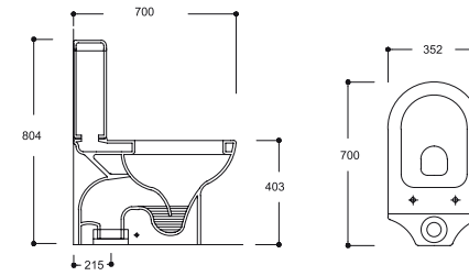
K001KLZ00 COMPACT KLOZET (ALT ÇIKIŞLI)
