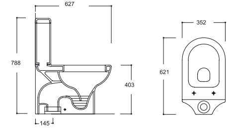
K007KLZ00 COMPACT KLOZET (ALT ÇIKIŞLI, KISA Q)
