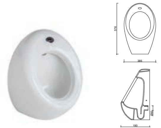
AR01PSR00 ARYA ANKASTRE FOTOSELLİ PİŞUVAR
